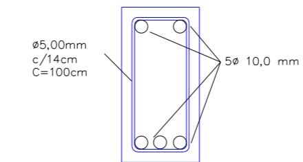
DETALHAMENTO SECÇÃO VIGAS SEM ESCALA
