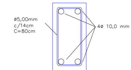
DETALHAMENTO SECÇÃO PILARES SEM ESCALA
