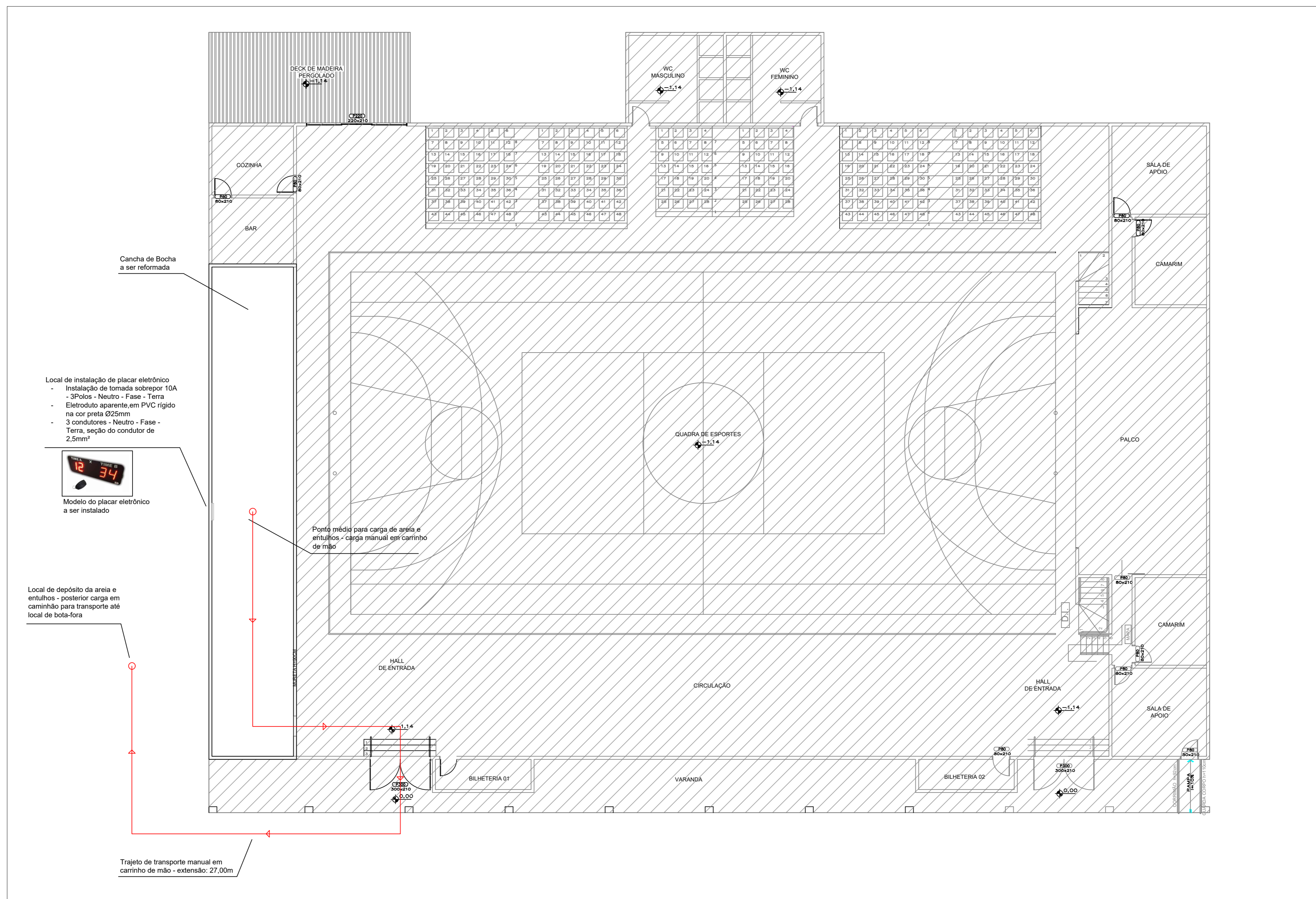
PLANTA BAIXA - SITUAÇÃO / LAYOUT ESC: 1/75
