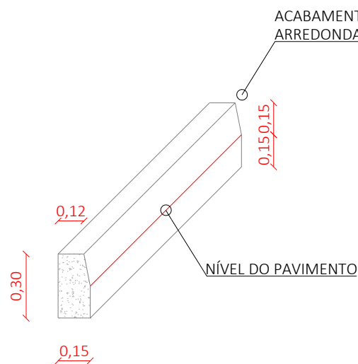
DETALHE MEIO-FIO ESC: 1/25
