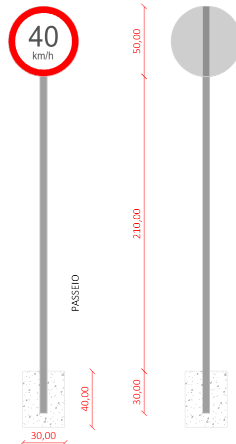
DETALHE PLACA DE SINALIZAÇÃO SEM ESCALA
