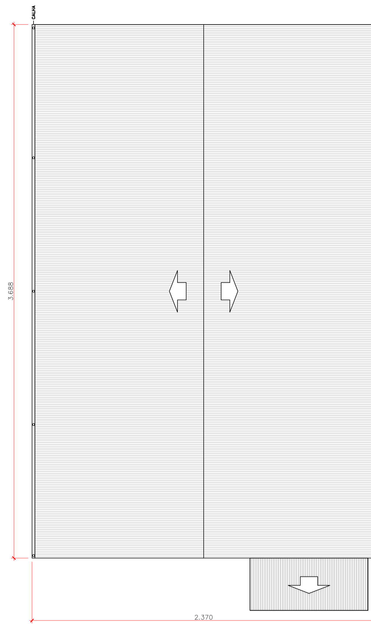
PLANTA DE COBERTURA - GINÁSIO JACINTA NUNES Esc. 1:150
