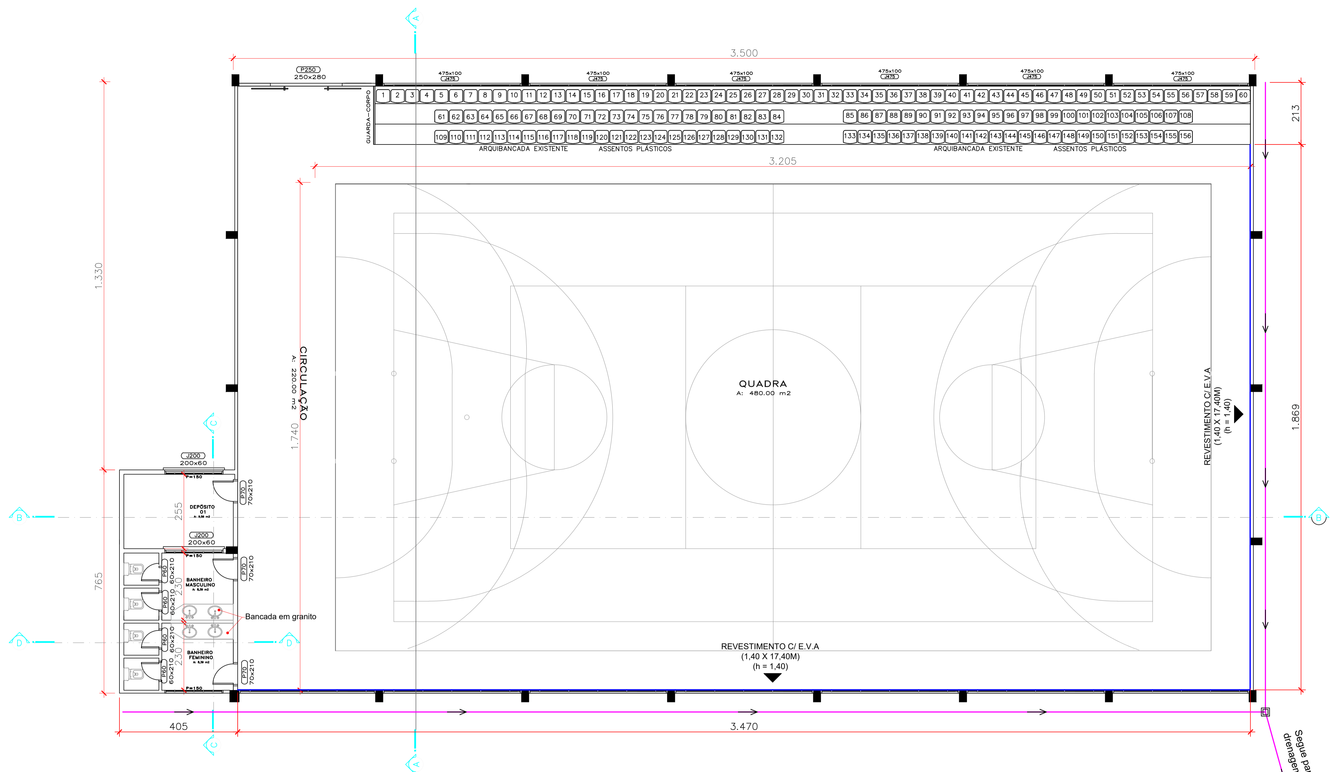
PLANTA BAIXA - GINÁSIO JACINTA NUNES Esc. 1:75
