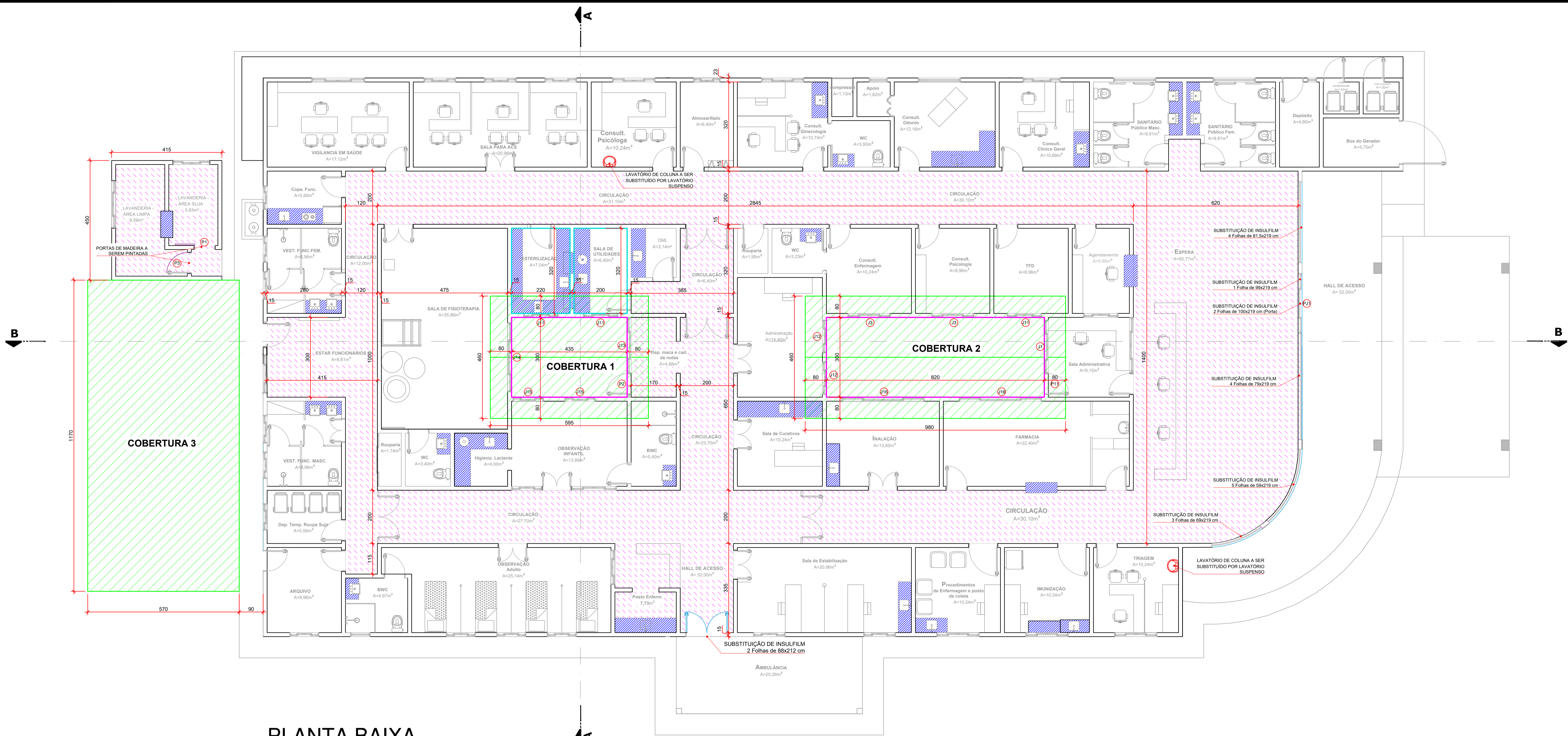
PLANTA BAIXA Esc. 1:75
