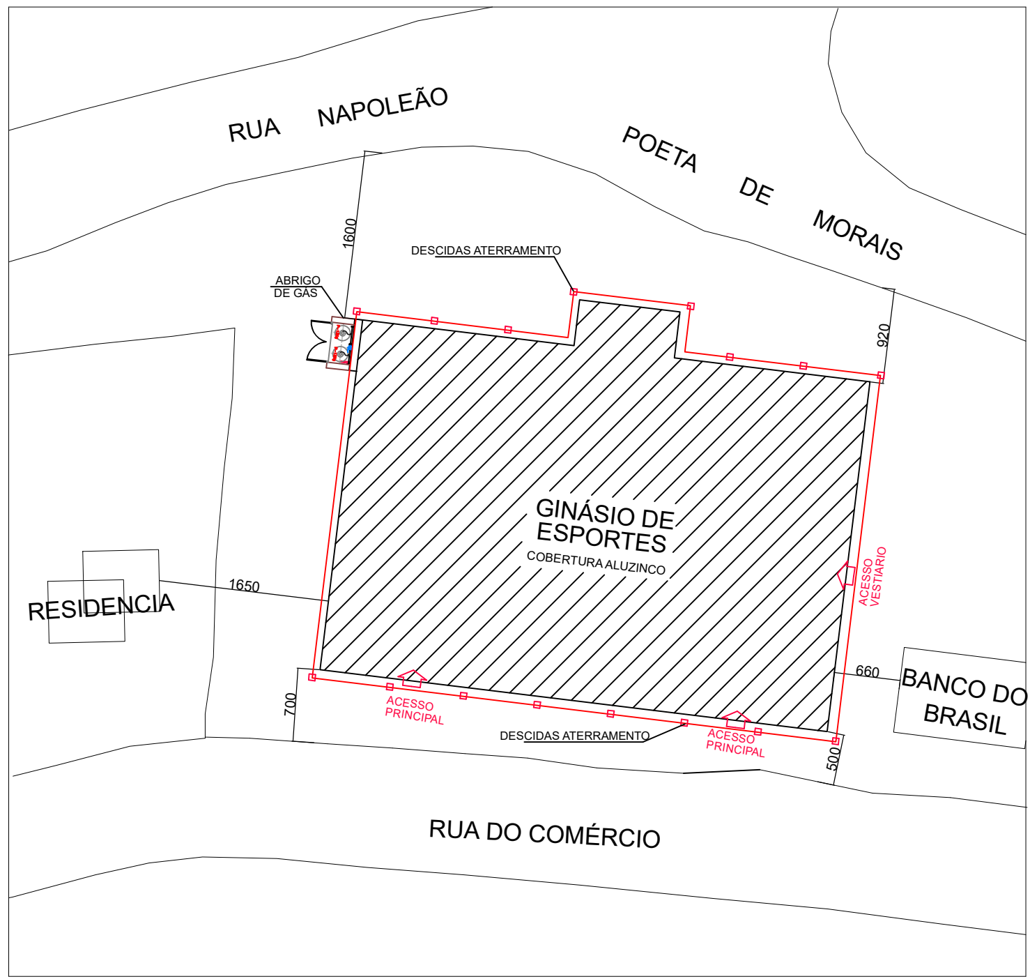
PLANTA DE SITUAÇÃO/LOCALIZAÇÃO Escala 1/500
