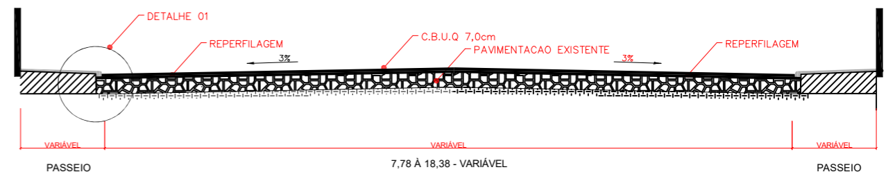
DETALHE 02 SOBRE CALÇAMENTO
