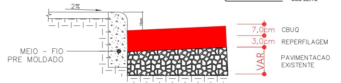
DETALHE 02 SOBRE CALÇAMENTO
