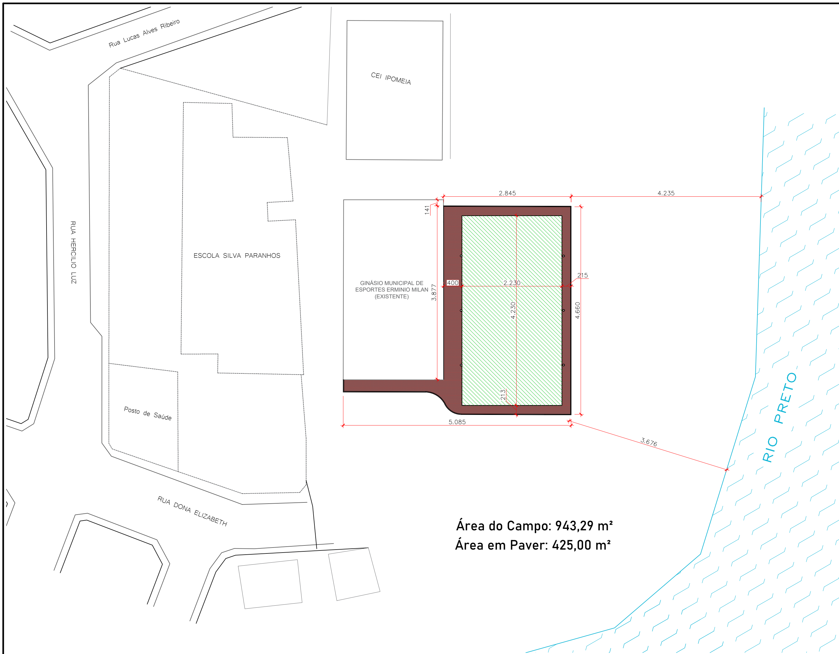
PLANTA DE LOCALIZAÇÃO Esc. 1:500
